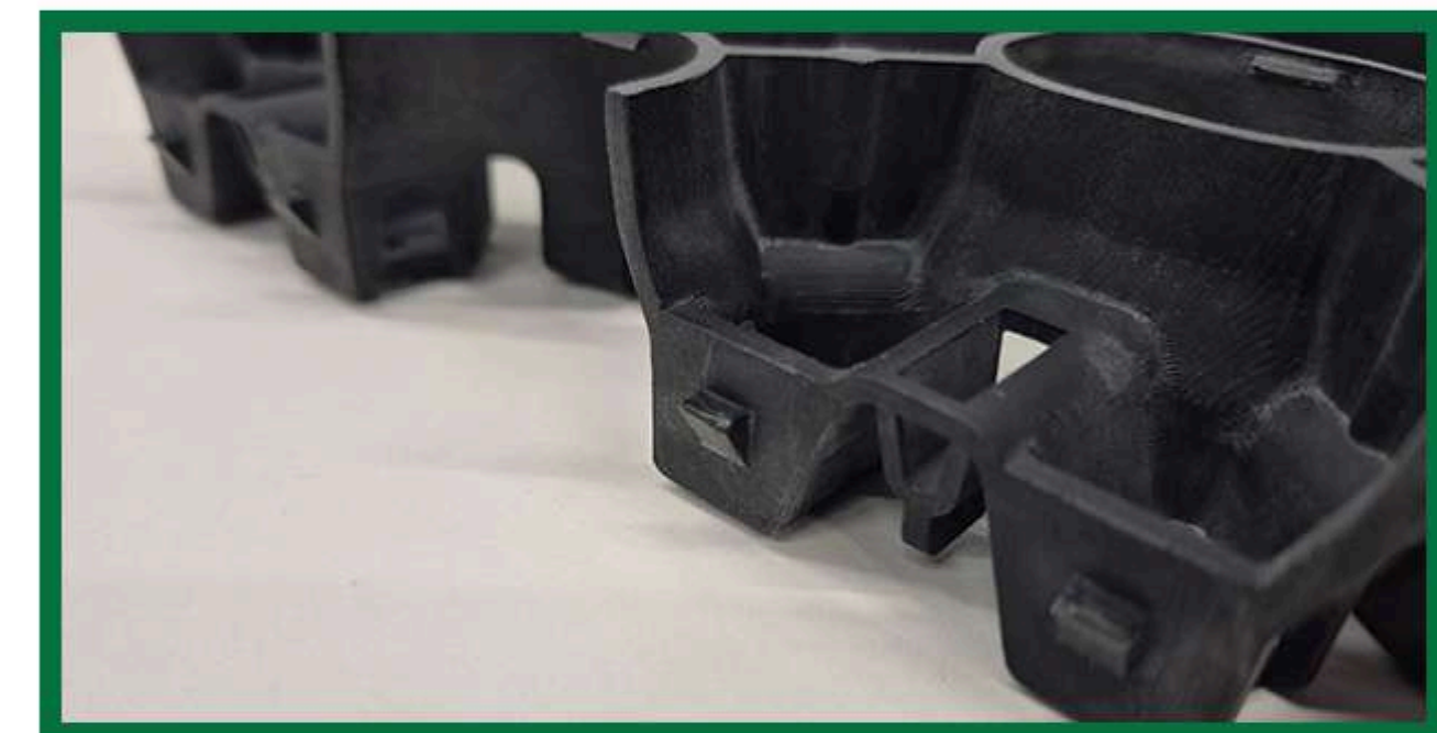
Male lugs
